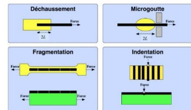
Tests d'adhésion fibre/matrice et couche mince/substrat
