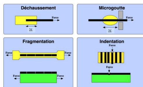
Tests d'adhésion fibre/matrice et couche mince/substrat
